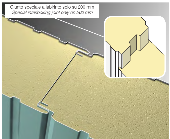
Calcoli effettuati su pannello con paramenti di acciaio 0,4 + 0,4 mm * (a 8 giorni da produzione / 8 days from production)
